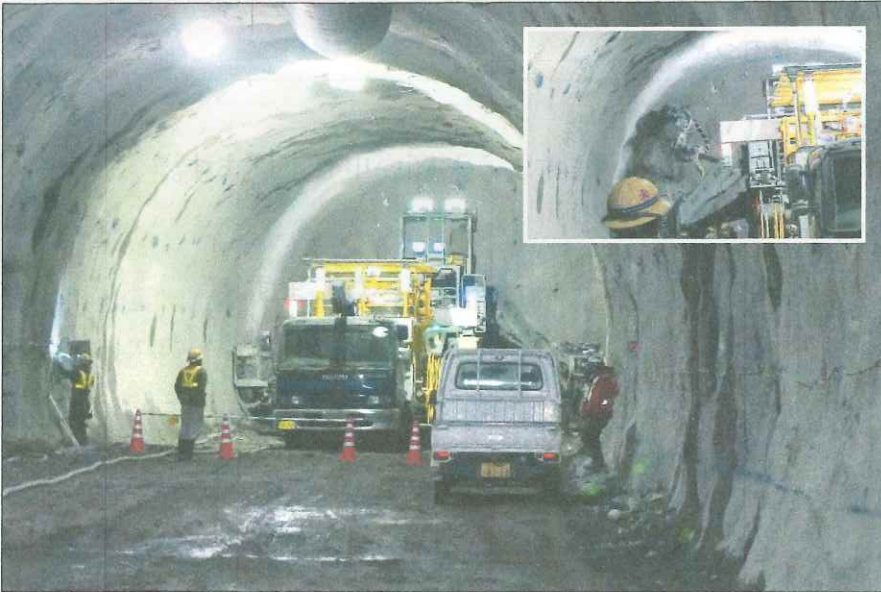
切羽部でドリルジャンボによる削孔
